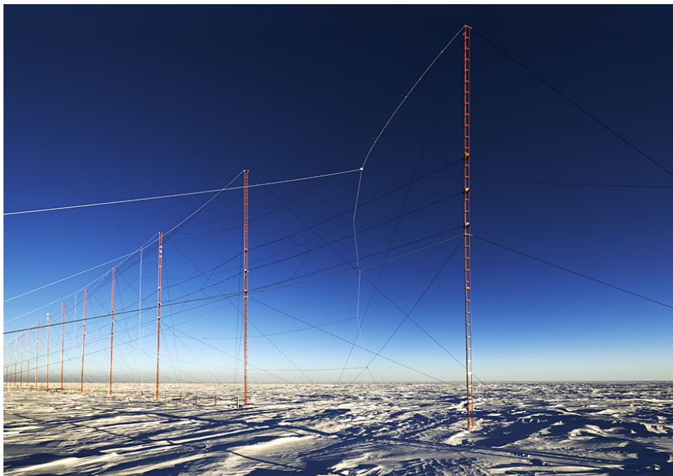
Rete SuperDARN presso la stazione Concordia
